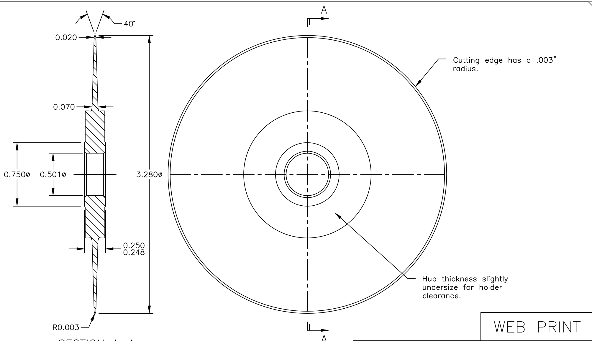
SECTION A-A
