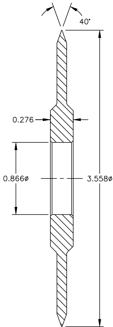
SECTION A-A
