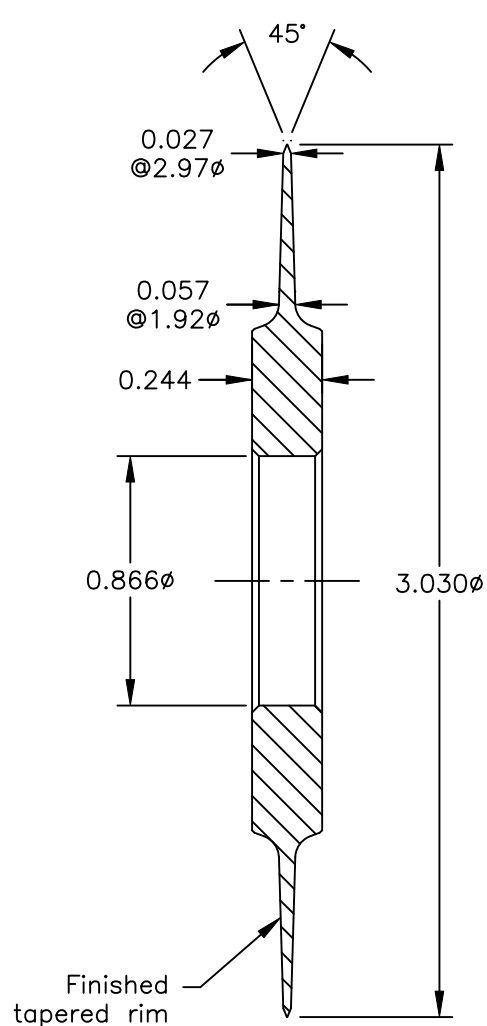
SECTION A-A
