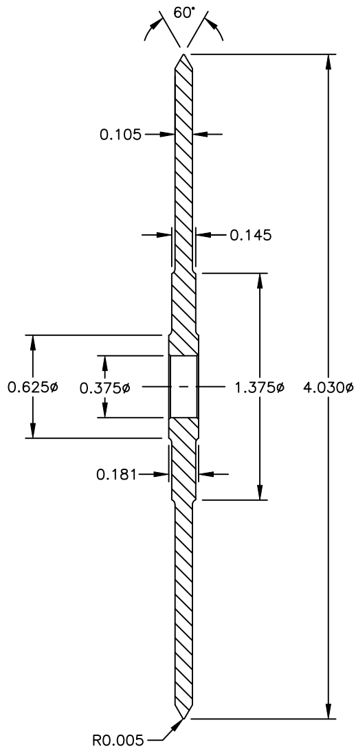
SECTION A-A
